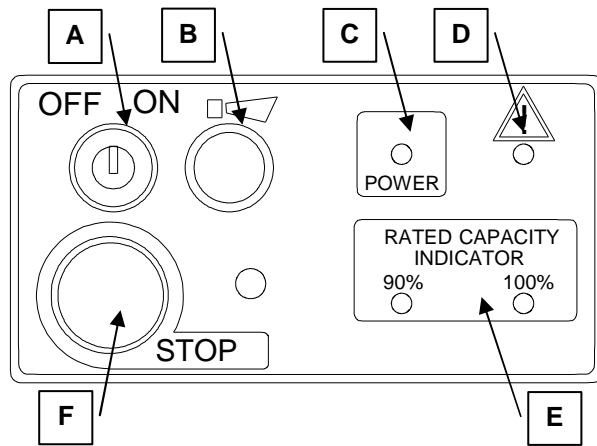
PANEL PRZY ZAWORZE Panel at control valve side
